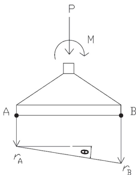
Figura 7 Determinação da rotação nas sapatas
