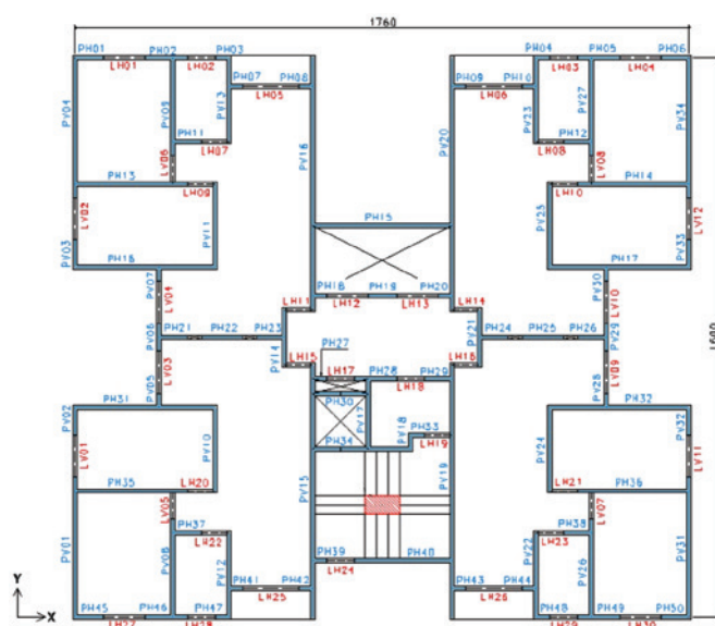
Figura 8 Planta baixa do edifício (Fonte: Braguim, 2013)
