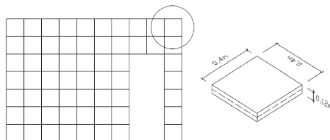
Figura 2 Discretização da parede em elementos de casca
