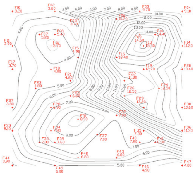
Figura 12 Curva de isorecalque do modelo CASCA RIG
