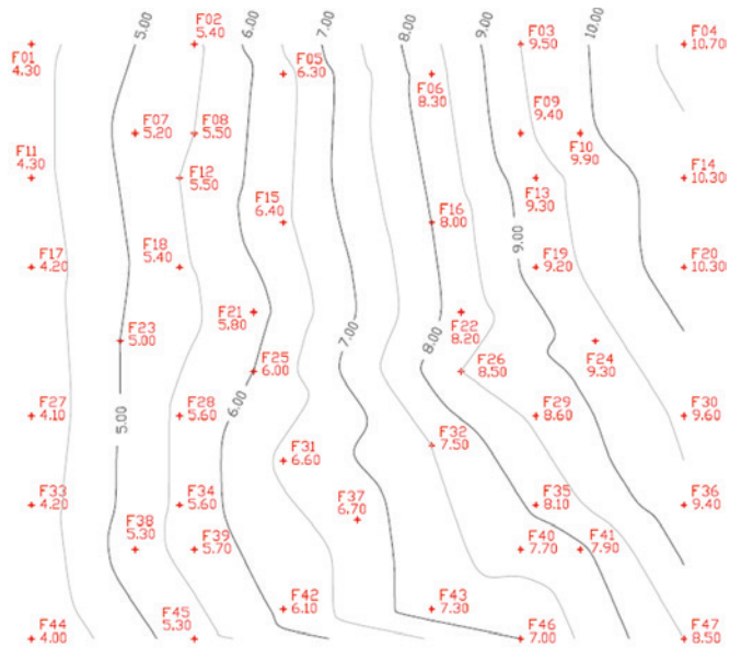
Figura 13 Curva de isorecalque do modelo CASCA ISE
